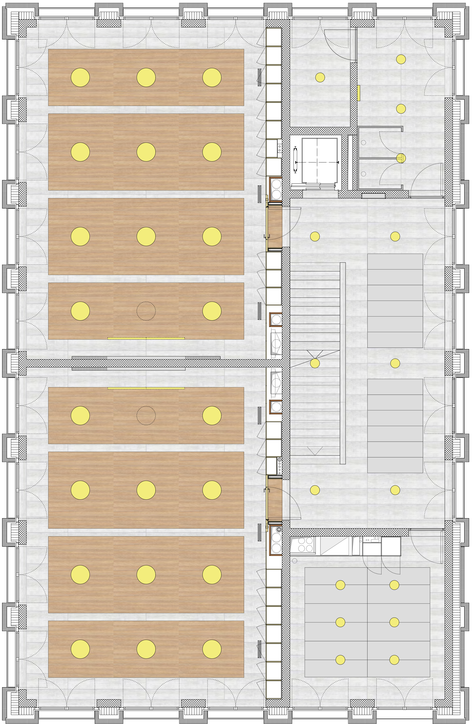
DECKENSPIEGEL OBERGESCHOSS
