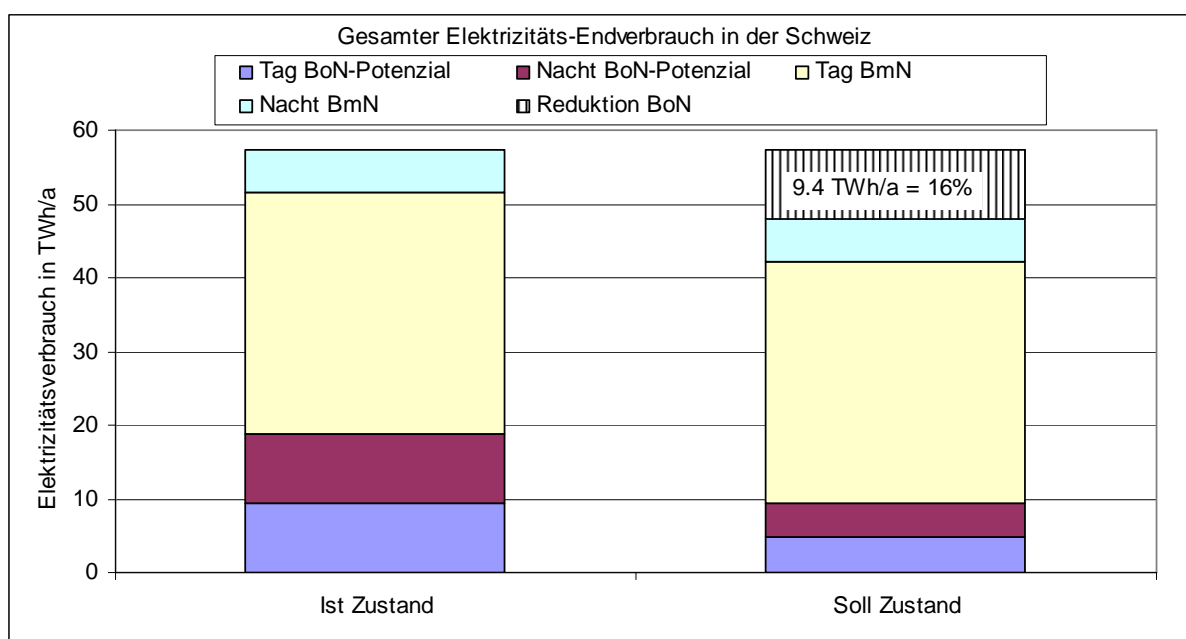
Bild 21: Gesamter elektrischer Endverbrauch: Abschätzung Anteil BoN
